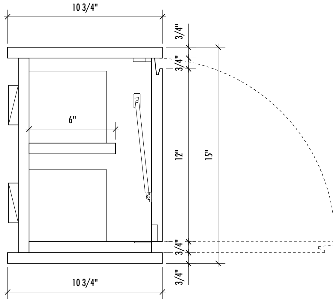
505 A.V. UNIT SECTION (TYP.) SCALE 3"=1'-0"
